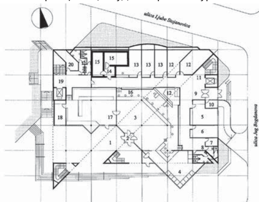
Основа приземља
