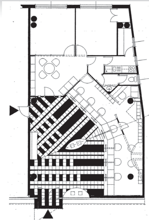
Основа
