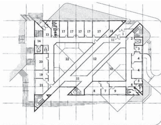
Основа првог спрата
