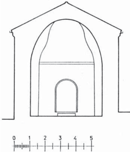
Св. Јован, попречни пресек
