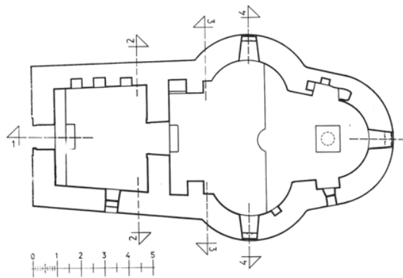
Св. Јован, основа
