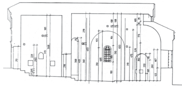
Св. Јован, подужни пресек
